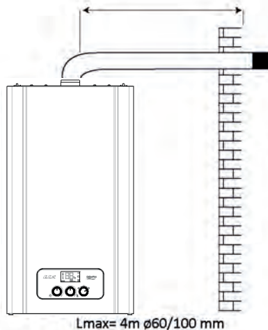
а) Пример дымохода с использованием одного 90^\circ отвода.
