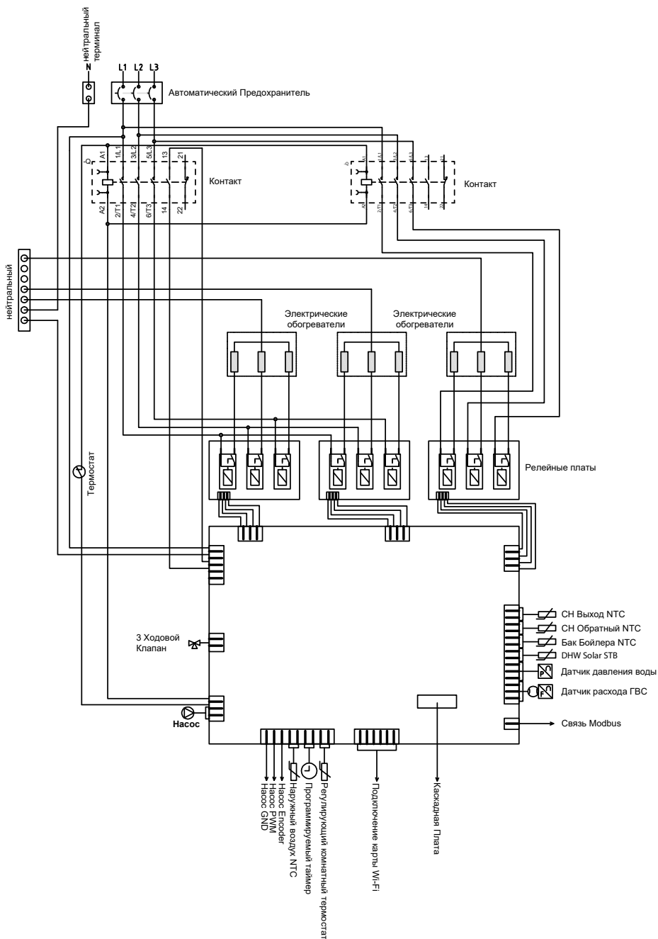
Рисунок 4. Arceus 27 кВт Схема Соединения
