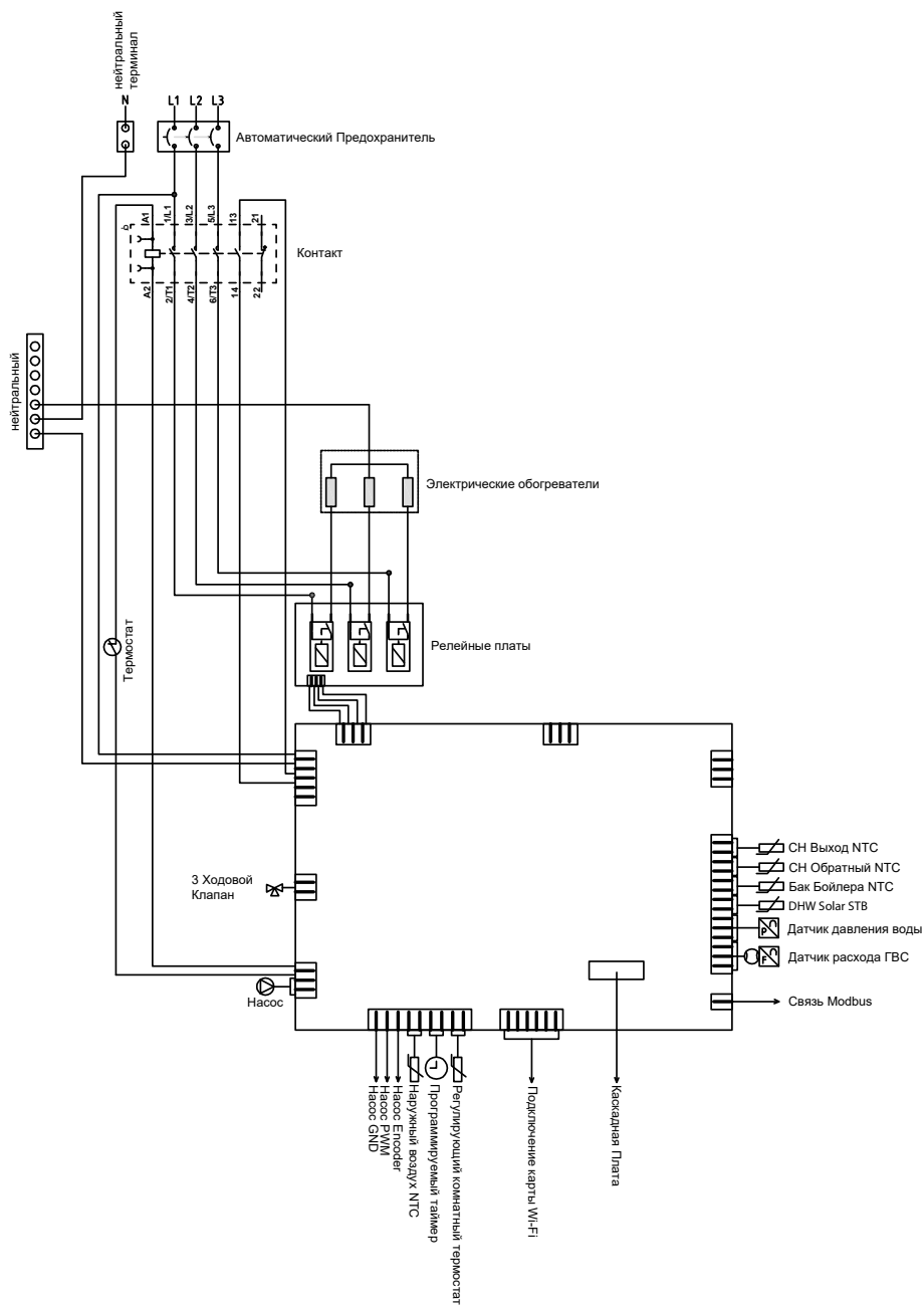
Рисунок 1. Arceus 6-9 кВт Схема Соединения
