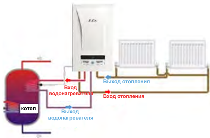
Рисунок 9. Схема подключения устройства ST.
