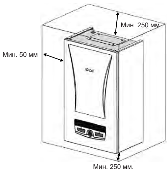
Рисунок 10. Необходимое пространство для установки устройства.
