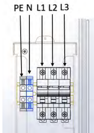
Рисунок 15. Входы электрического подключения устройства.
